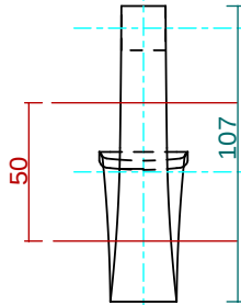
唐草頭部詳細 1:3
