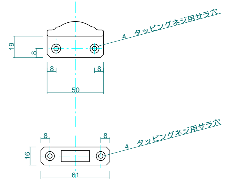
壁付BPL詳細 1:2
