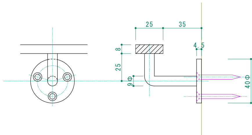
壁付けサポート詳細 scale:1:2
